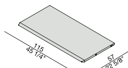
Ripiano 120 Legno Shelf 120 Wood
