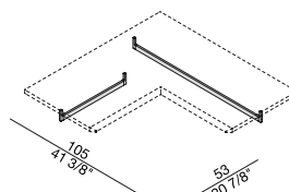
Appenderia angolare Corner Hanging bar
