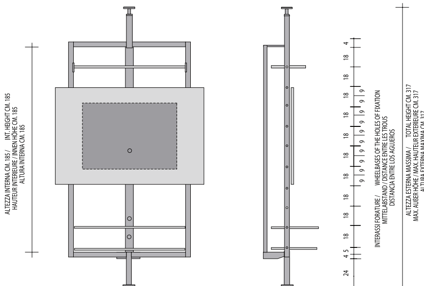
COMP. U36
