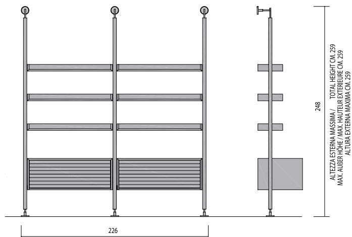
COMP. U52
