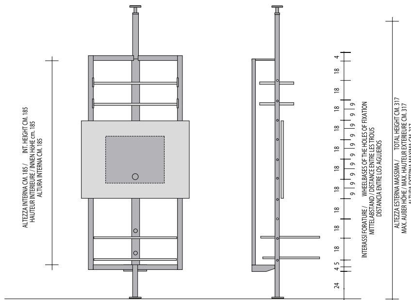
COMP. U43
