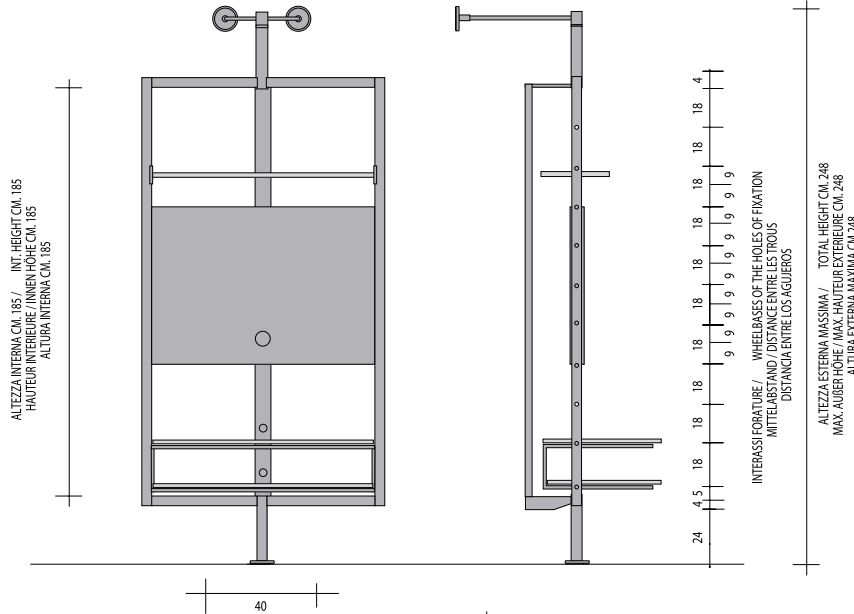
COMP. U28
