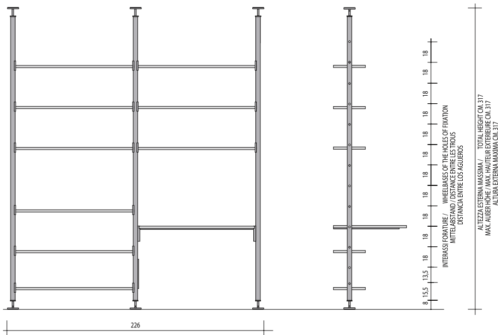
COMP. U33
