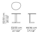
Кумо 53 high Ширина: 53см Глубина: 44см Высота: 52/55см
