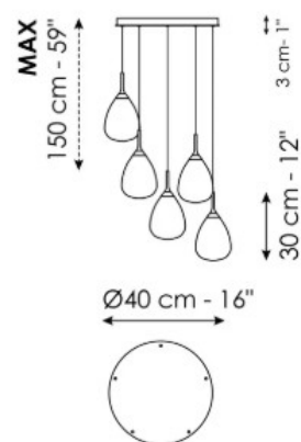
Gocce - 5 lights Ширина: 40cm Глубина: 40cm Высота: 30cm
