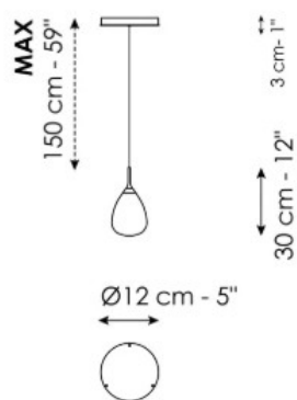
Gocce - 1 light Ширина: 12cm Глубина: 12cm Высота: 30cm
