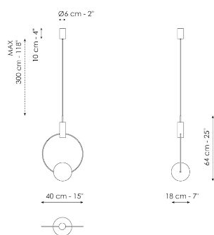
Keshi - 1 light Ширина: 40cm Глубина: 18cm Высота: 64cm
