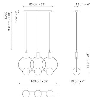
Keshi - 3 lights linear Ширина: 100cm Глубина: 18cm Высота: 64cm
