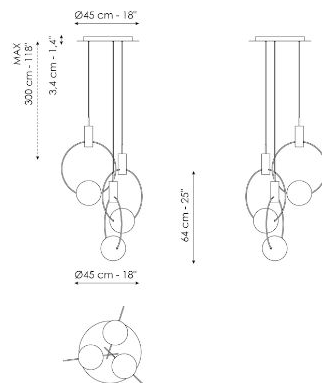
Keshi - 3 lights casual Ширина: 40cm Глубина: 48cm Высота: 64cm
