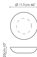
Big planet
