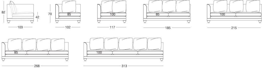
Terminali Sx / End unit L.H. / Боковые секции Л
